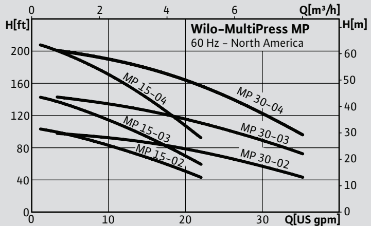
Wilo MP Non Self-Priming
